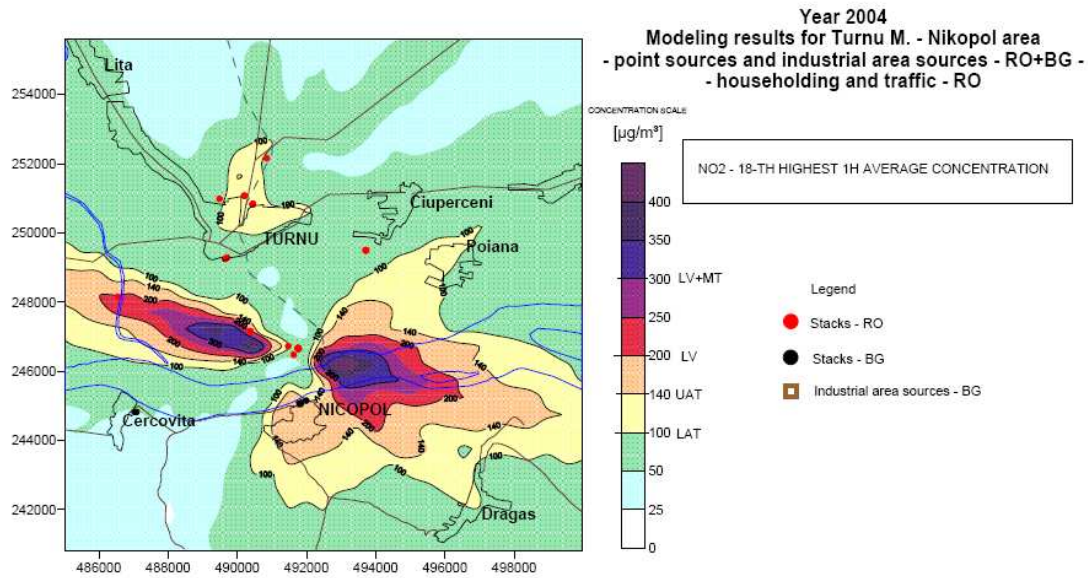
Figura 21. A 18-a cea mai mare concentrație orară modelată pentru NO 2 în Turnu Măgurele în 2004. Unități \mu\text{g}\cdot\text{m}^{-3} .
