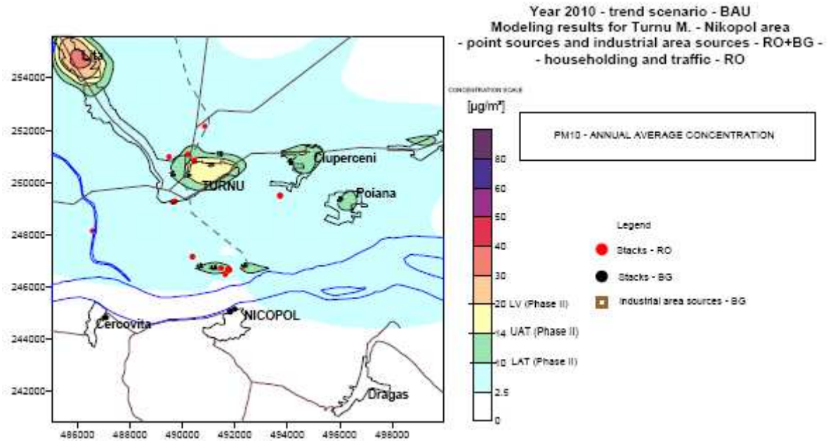
Figura 20. Modelarea concentrației medii anuale de PM 10 în Turnu Măgurele în 2010. Unități µg.m -3 .
