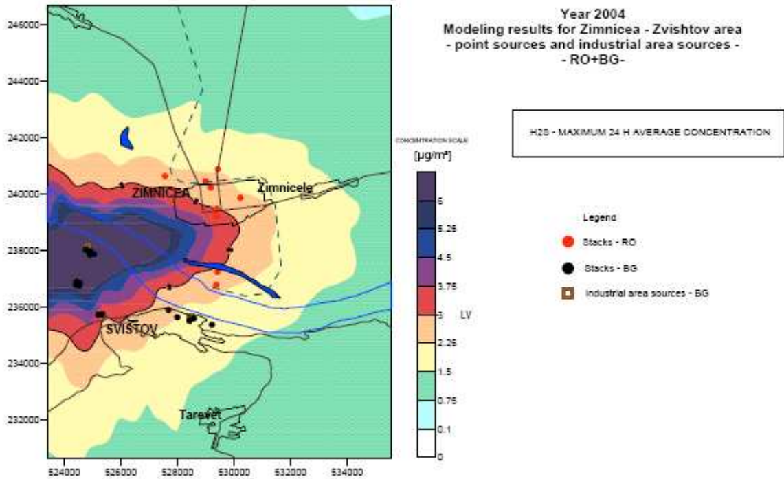
Figura 39. Modelarea concentrației maxime zilnice de H 2 S în Zimnicea în 2004. Unități µg.m -3 .
